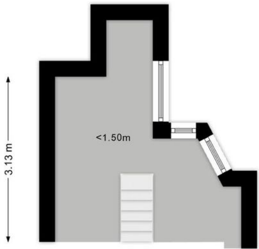
Tweede verdieping, Wagendwarsstraat 58 te Utrecht. Deze plattegronden zijn opgemaakt voor indicatieve doeleinden. Hieraan kunnen geen rechten worden ontleend.
