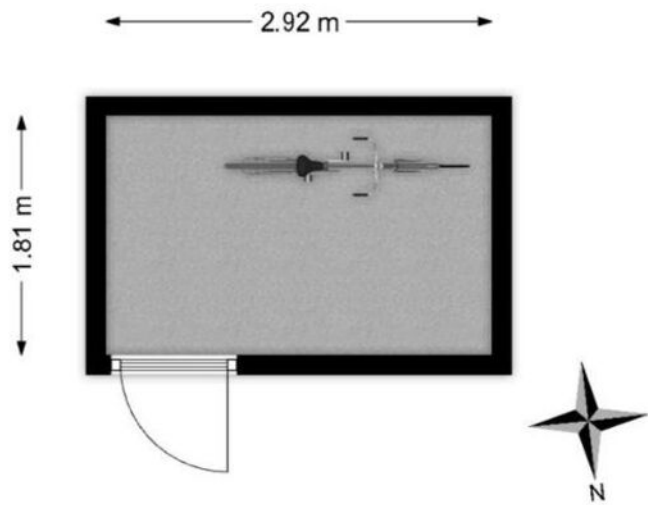
Berging, Louis Armstronglaan 568 te Utrecht Deze plattegronden zijn opgemaakt voor indicatieve doeleinden. Hieraan kunnen geen rechten worden ontleend.
